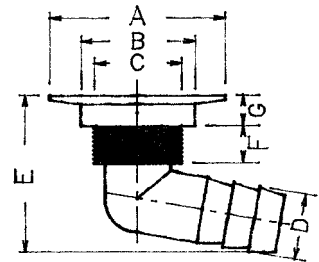
3997 - Elbow
