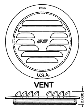
8475 - 8" Vent
